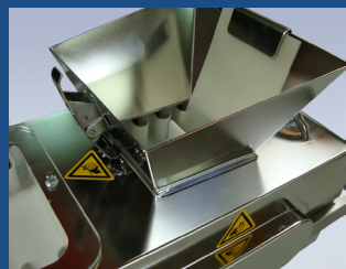
配有快速安装张紧轮的 装料漏斗
